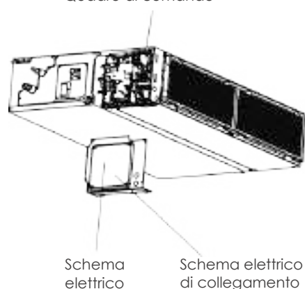
Quadro di comando
