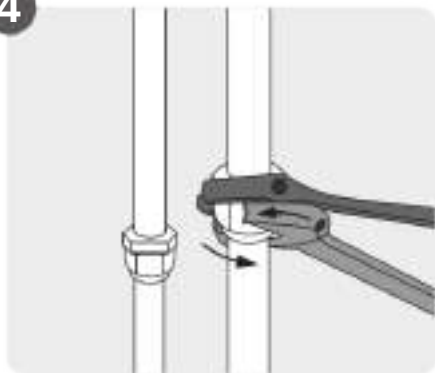
Collegare i tubi del refrigerante
