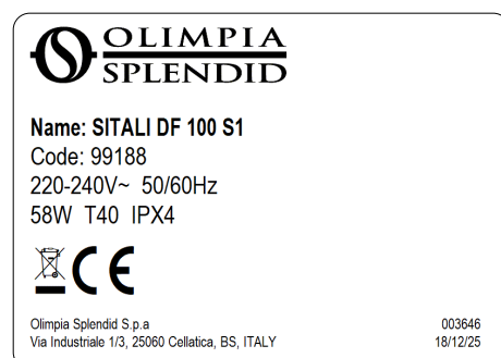
Fig. 2.c Etichetta dati
