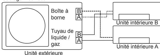
Câblage incorrect
