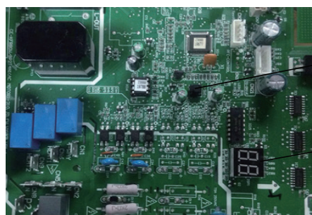
Correcto
