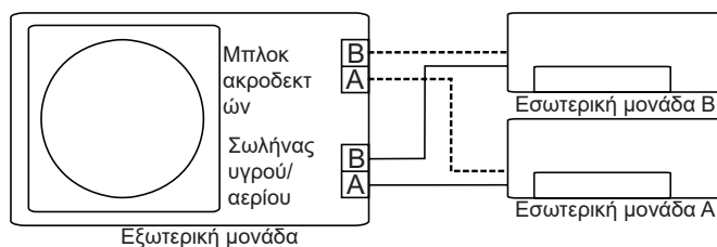
Λανθασμένη καλωδίωση
