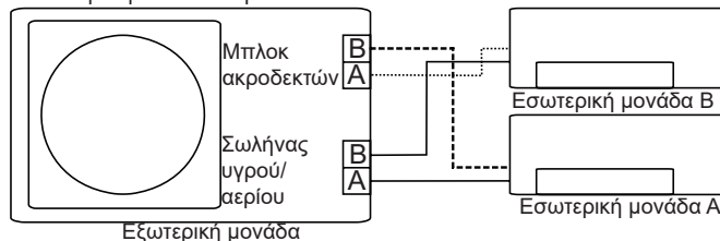
Λανθασμένη καλωδίωση
